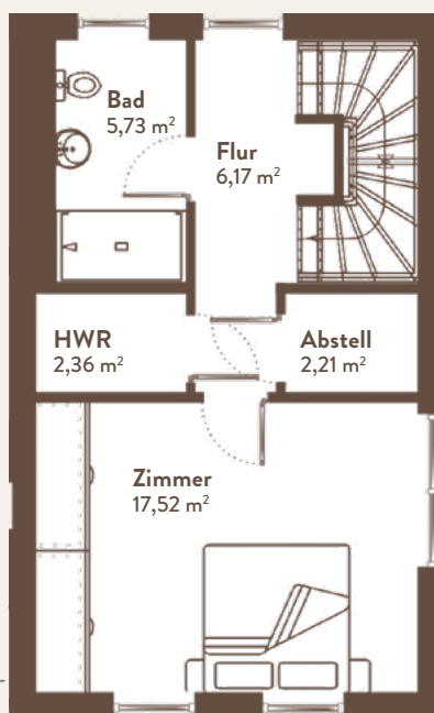
OBERGESCHOSS
